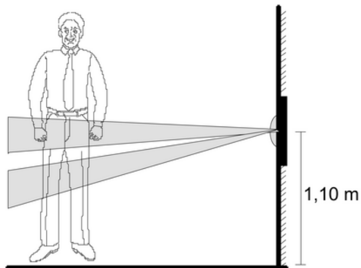
Bild 8: Erfassungsebenen
