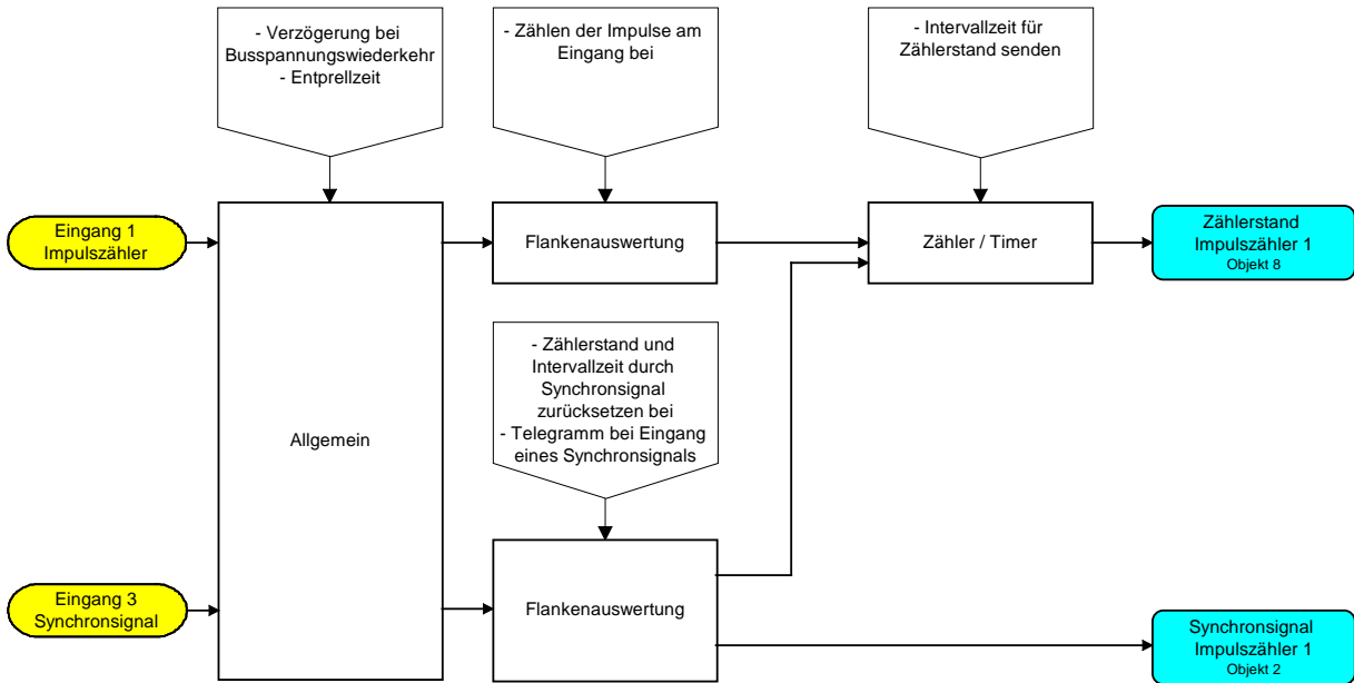
Funktionsschaltbild (für Binäreingang / z. B. Eingang 1 Funktion "Impulszähler")
