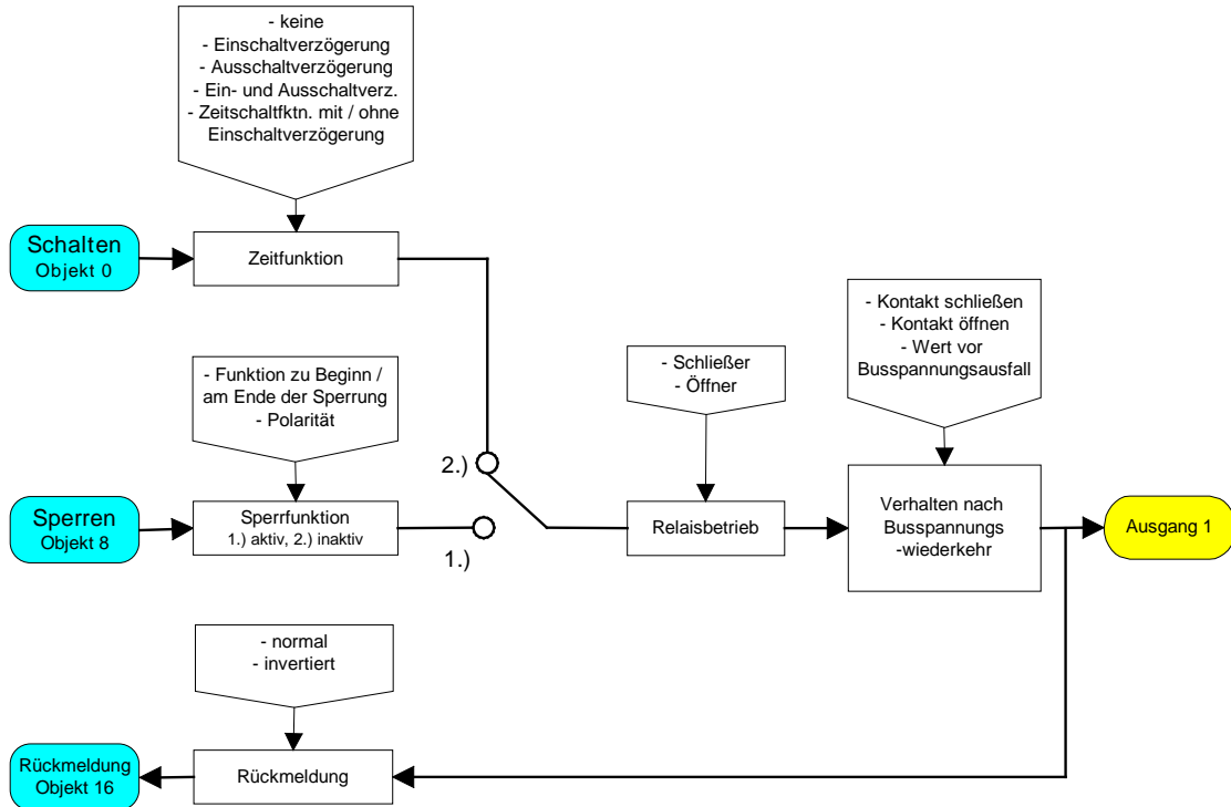
Funktionsschaltbild (für Schaltausgänge / z. B. Ausgang 1 mit der Zusatzfunktion "Sperrobject")
