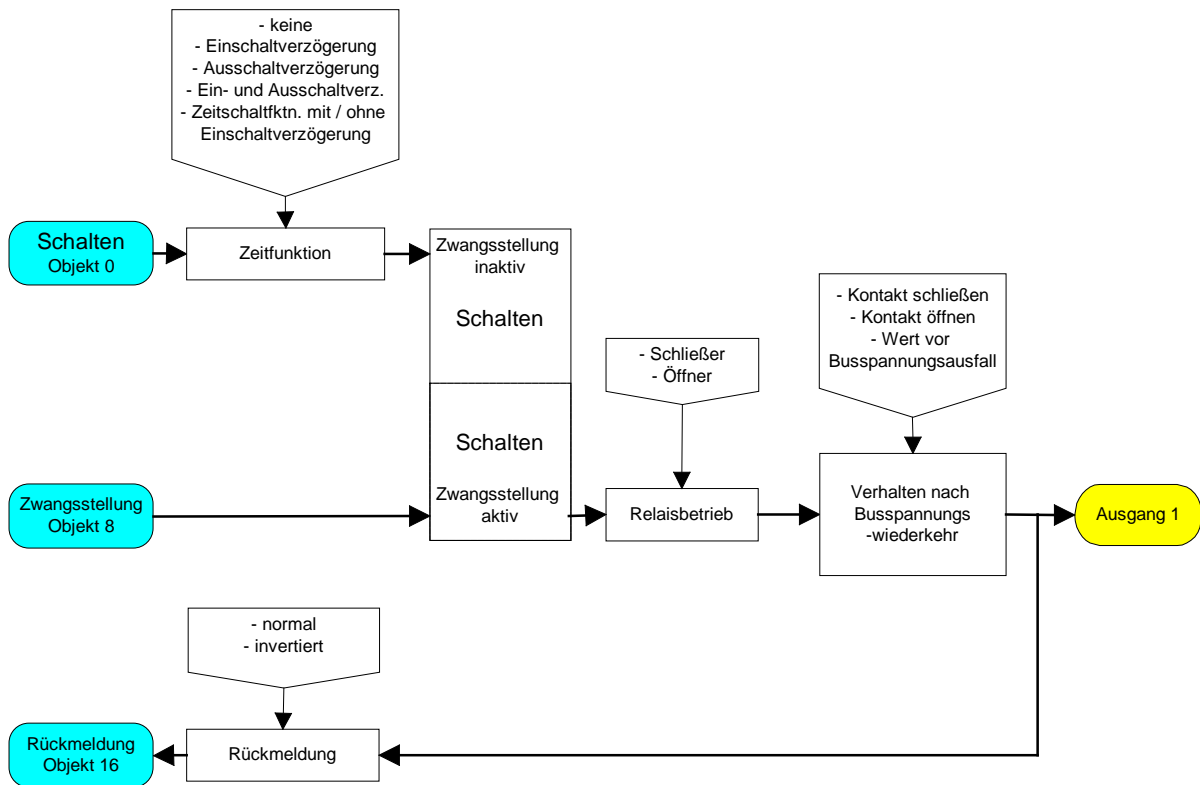
Funktionsschaltbild (für Schaltausgänge / z. B. Ausgang 1 mit der Zusatzfunktion "Zwangsstellungsobject")
