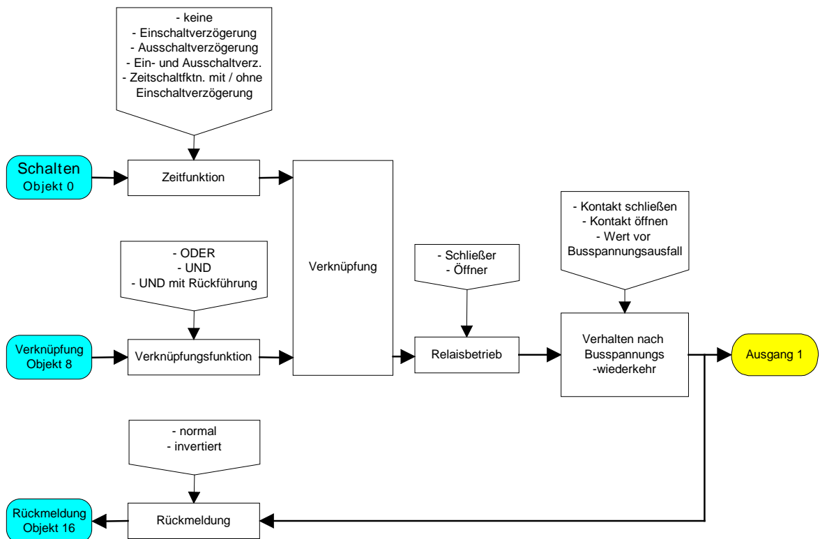
Funktionsschaltbild (für Schaltausgänge / z. B. Ausgang 1 mit der Zusatzfunktion "Verknüpfungsobjekt")
