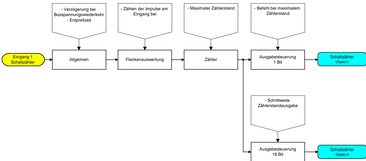
Funktionsschaltbild (für Binäreingang / z. B. Eingang 1 Funktion "Schaltzähler")
