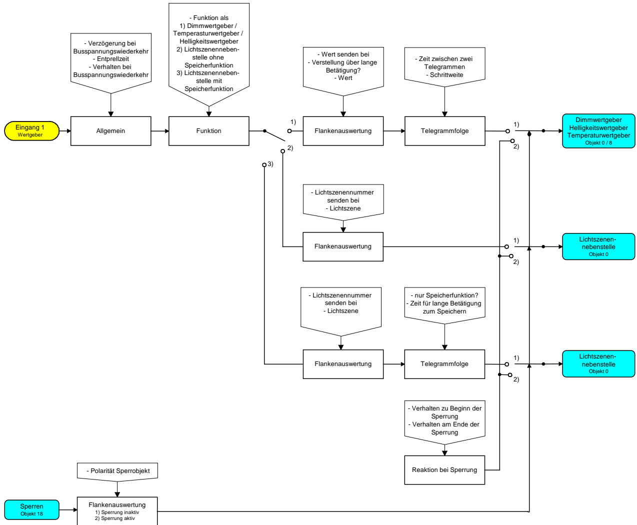
Funktionsschaltbild (für Binäreingang / z. B. Eingang 1 Funktion "Wertgeber")
