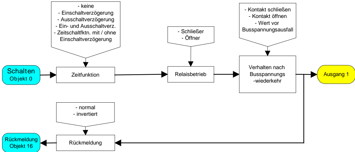
Funktionsschaltbild (für Schaltausgänge / z. B. Ausgang 1 ohne Zusatzfunktion)
