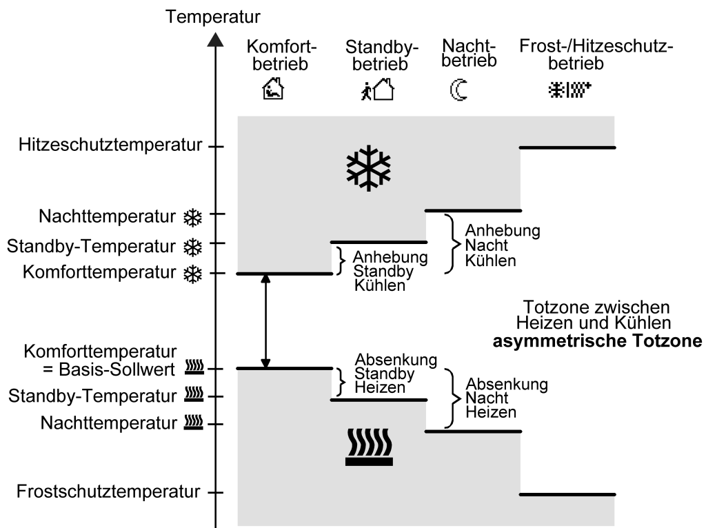
Bild 30: Solltemperaturen in der Betriebsart "Heizen und Kühlen" mit asymmetrischer Totzone
