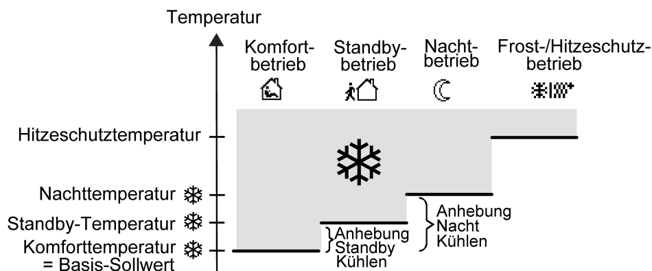
Bild 27: Solltemperaturen in der Betriebsart "Kühlen"
