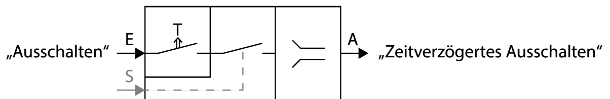
Bild 56: Schematische Darstellung "Zeitverzögert Ausschalten"
