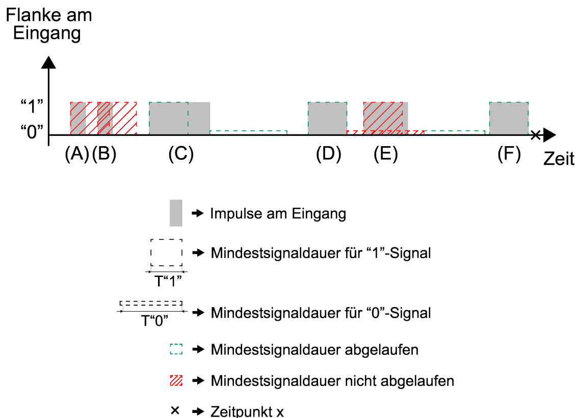
Bild 53: Beispiel zur Einstellung der Mindestsignaldauer
