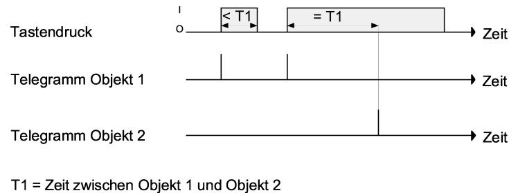
Bild 49: Beispiel zum Bedienkonzept "Objekt 1 und Objekt 2"
