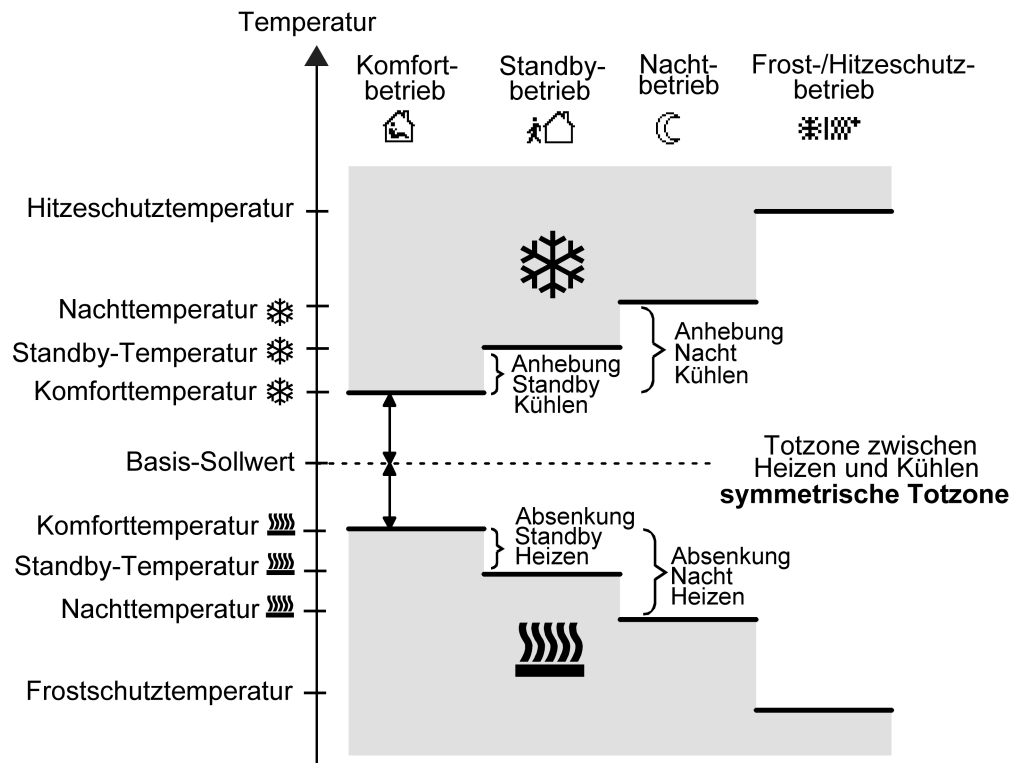
Bild 29: Solltemperaturen in der Betriebsart "Heizen und Kühlen" mit symmetrischer Totzone
