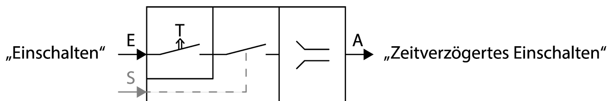
Bild 55: Schematische Darstellung "Zeitverzögert Einschalten"
