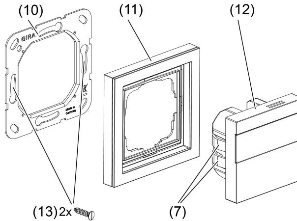
Bild 8: Gerät montieren
