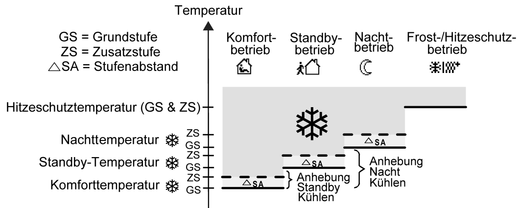
Bild 28: Solltemperaturen in der Betriebsart "Grund- und Zusatzkühlen"
