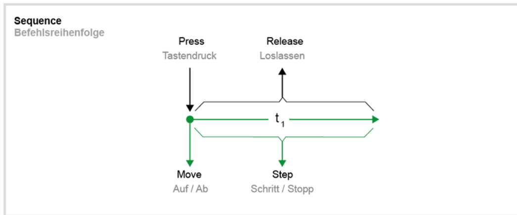
Bild 45: Bedienkonzept "Auf/Ab – Schritt"
