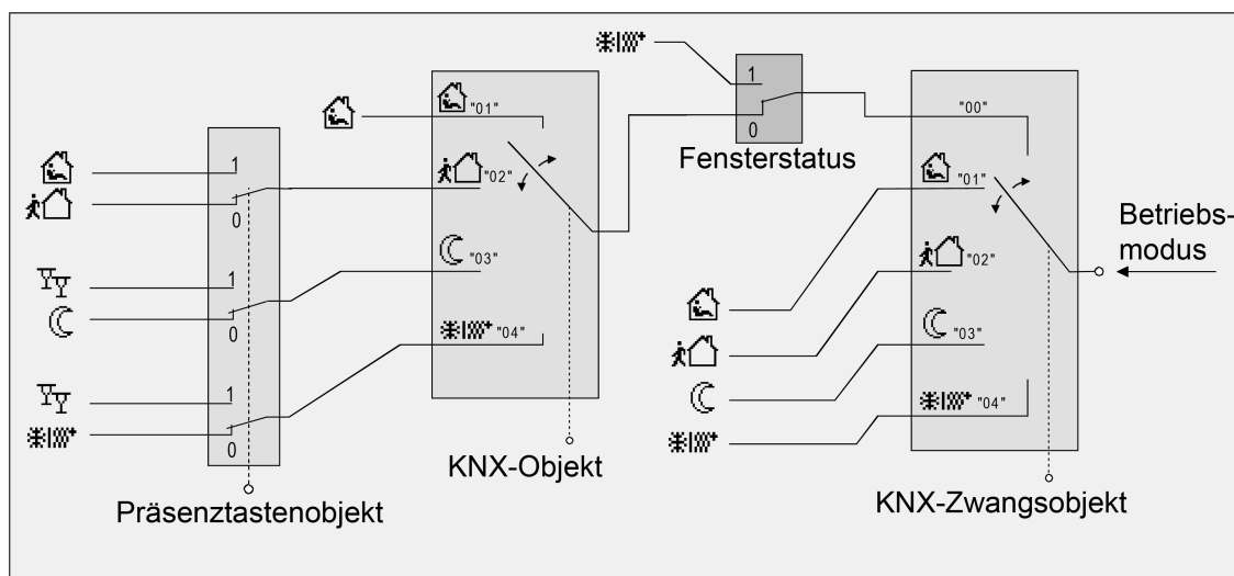
Bild 23: Betriebsmodusumschaltung durch KNX Objekt mit Präsenztaste
