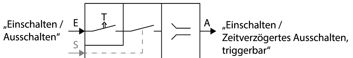
Bild 58: Schematische Darstellung "Treppenhausfunktion"
