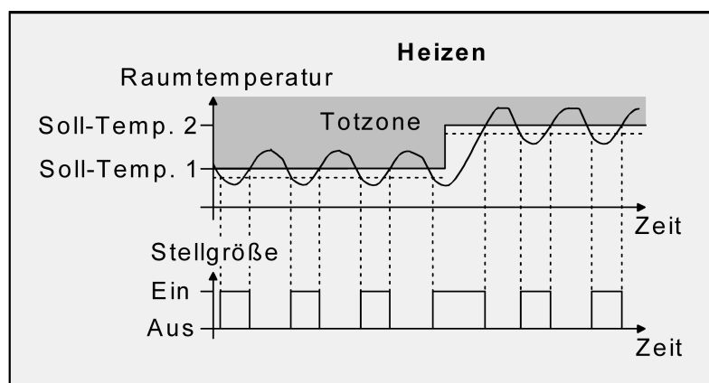
Bild 20: 2-Punkt-Regelung für Mischbetriebsart "Heizen und Kühlen" bei aktivem Heizbetrieb
