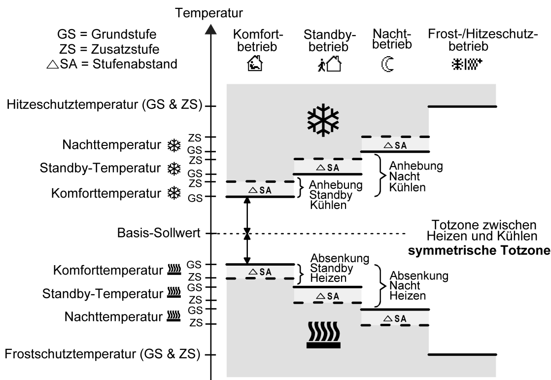
Bild 31: Solltemperaturen in der Betriebsart "Grund- und Zusatzheizen und -kühlen" mit symmetrischer Totzone
