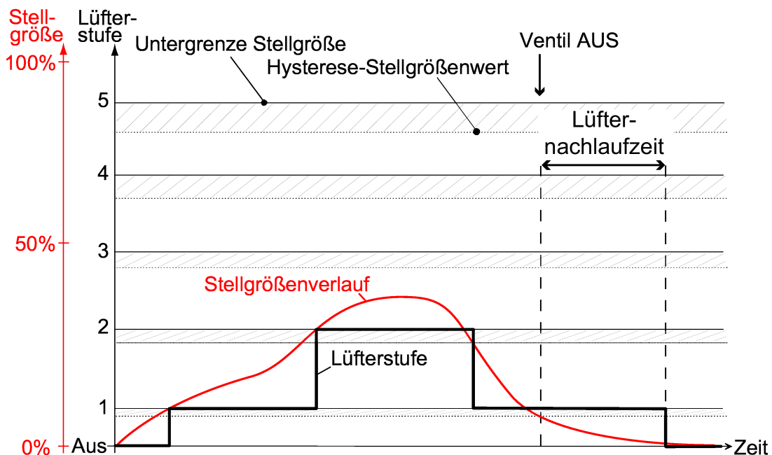
Bild 36: Vereinfachtes Stellgrößendiagramm zur Verdeutlichung einer Lüfterstufenumschaltung (aktive Lüfterstufe) unter Berücksichtigung einer Nachlaufzeit
