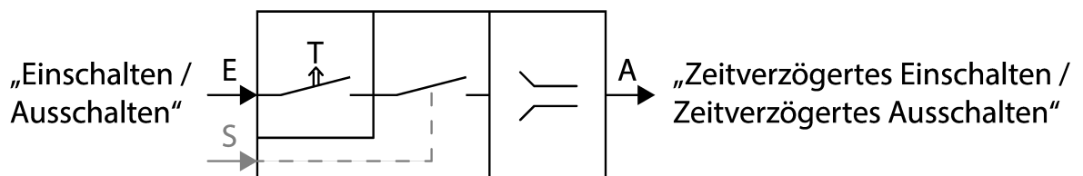
Bild 57: Schematische Darstellung "Zeitverzögert Ein- und Ausschalten"
