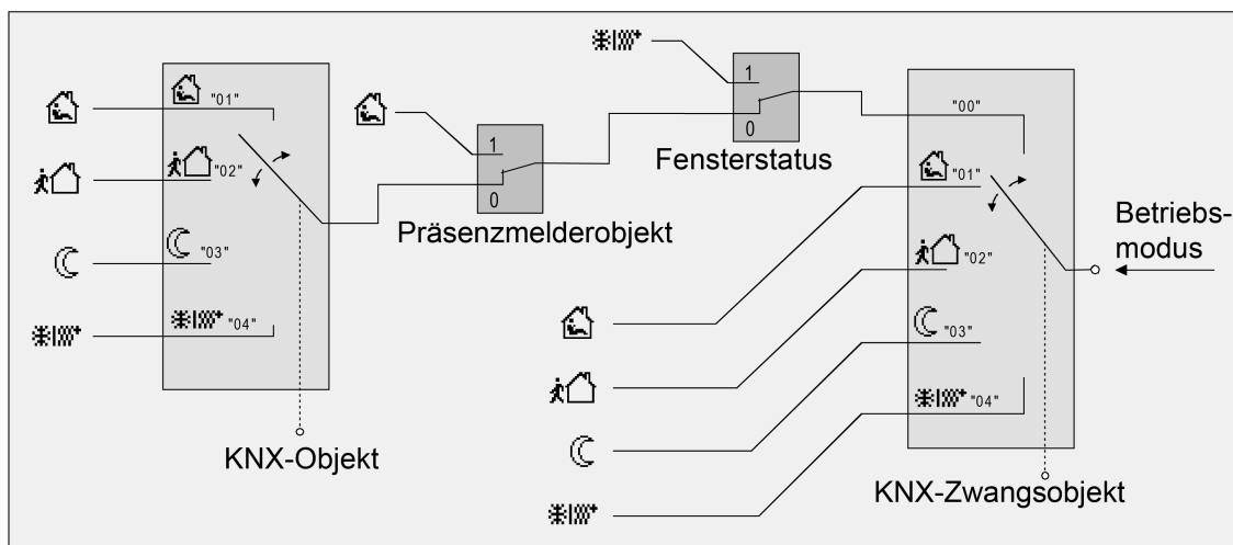
Bild 24: Betriebsmodusumschaltung durch KNX Objekt mit Präsenzmelder
