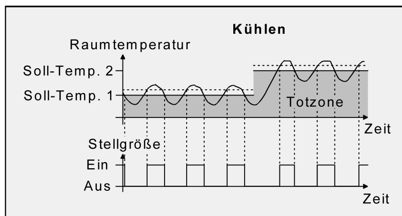
Bild 21: 2-Punkt-Regelung für Mischbetriebsart "Heizen und Kühlen" bei aktivem Kühlbetrieb
