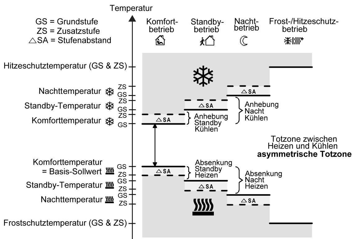
Bild 32: Solltemperaturen in der Betriebsart "Grund- und Zusatzheizen und -kühlen" mit asymmetrischer Totzone
