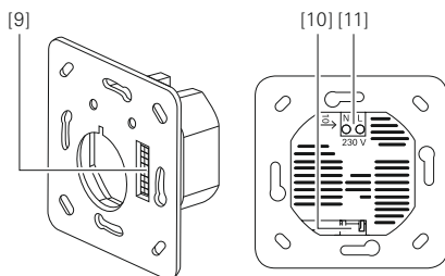
III. 3 Innfelt tilkoblingsmodul 230 V
