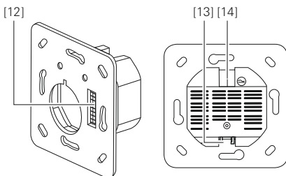
III. 4 Innfelt tilkoblingsmodul 24 V
