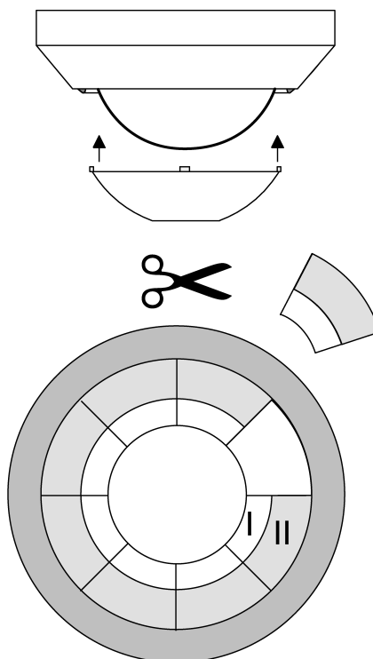
Afbeelding 11: Opsteekplaat
