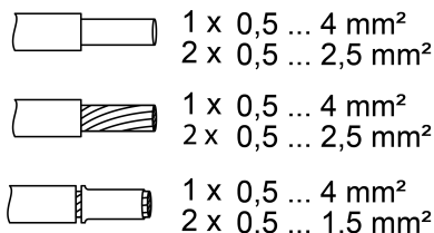
рисунок 4: Сечение провода под клемму
