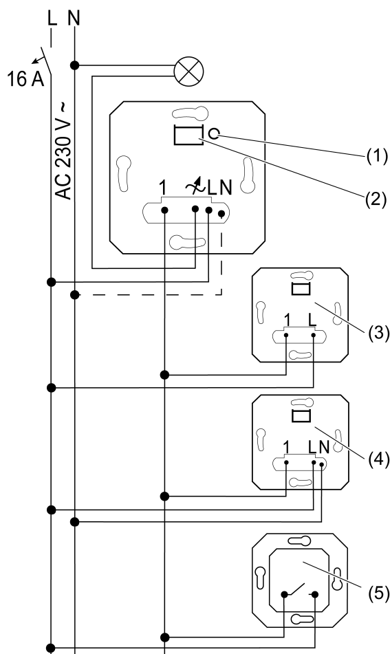
рисунок 1: Схема подключения с опциональными дополнительными узлами
