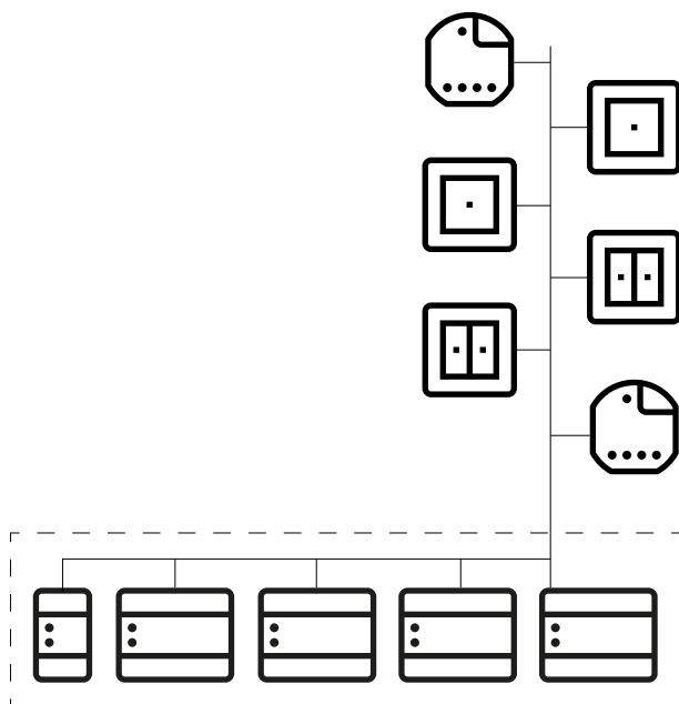
Linear wiring
