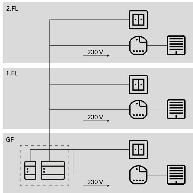
Decentrale installatie van de actuatoren
