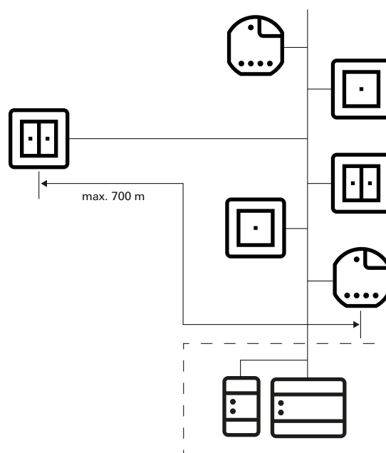
Afstand van twee willekeurige deelnemers: max. 700 m
