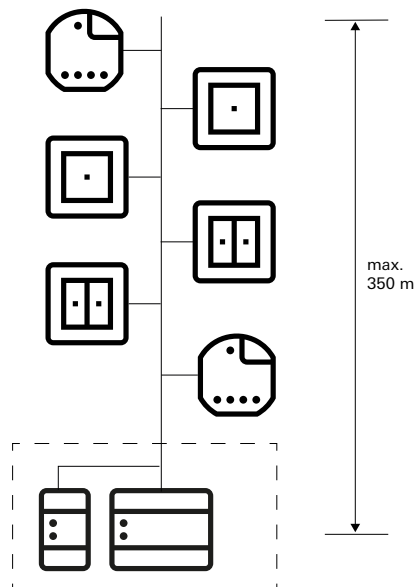
Afstand voedingsspanning – Deelnemers: max. 350 m
