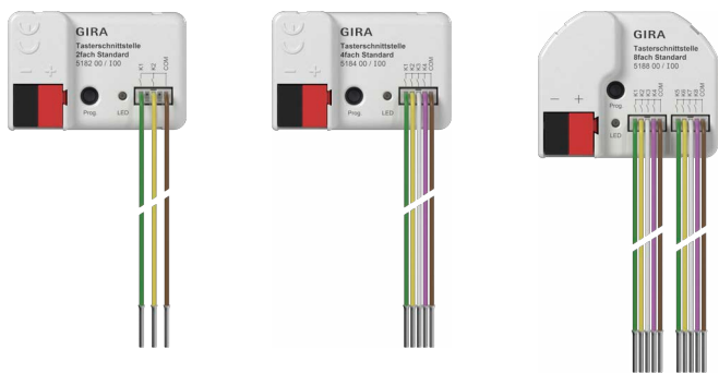
Artikelnr. 5182 00, 5184 00, 5188 00
