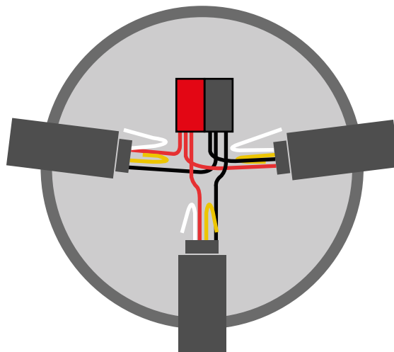
Aansluiting van de busdeelnemers
