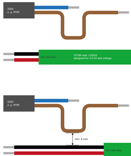
Afstand busleiding naar netleiding
